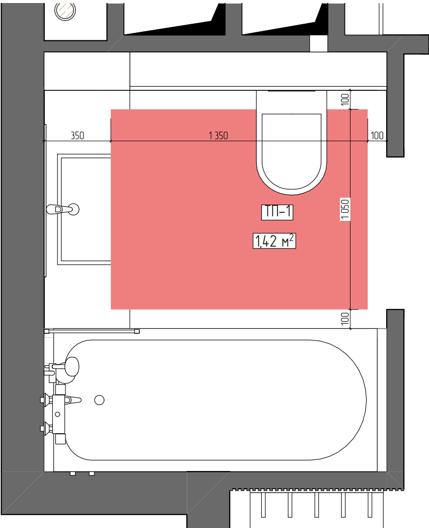
План теплого пола 1:20
