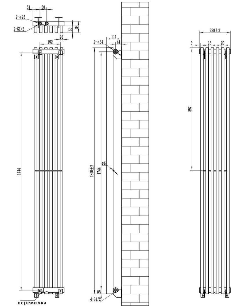
Трубчатый стальной радиатор отопления Sabron
