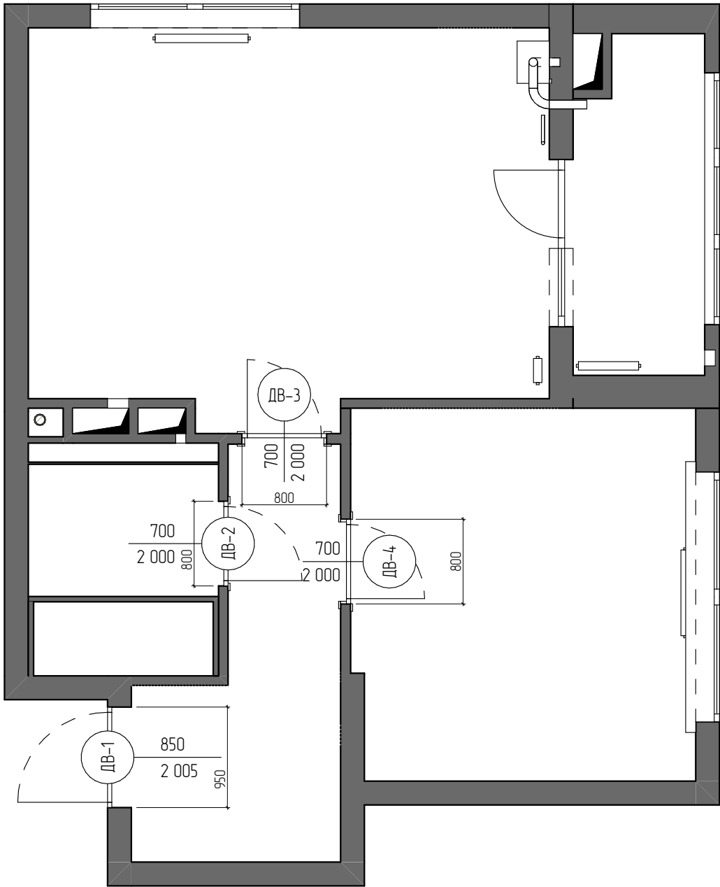
План дверей
