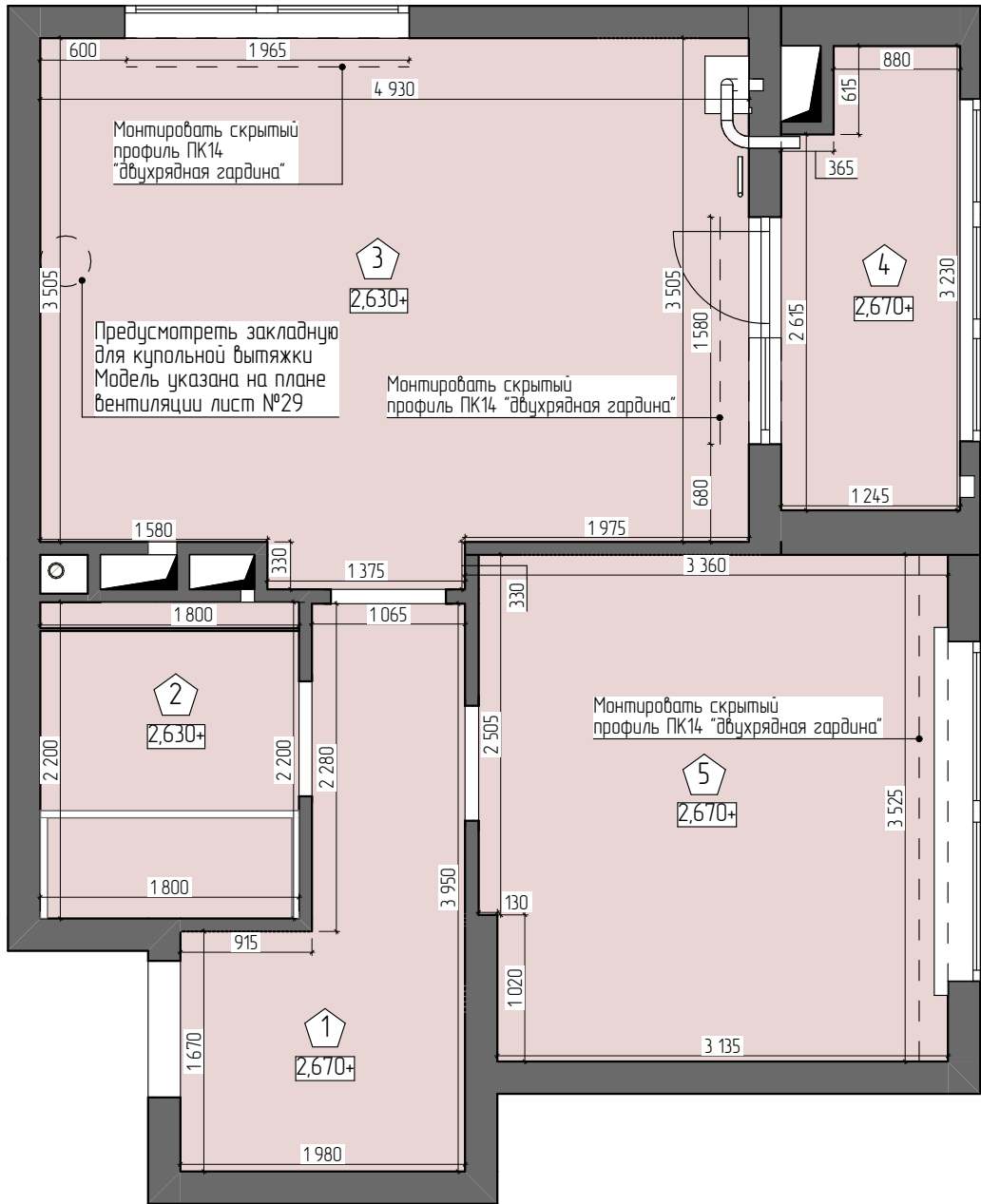
План потолков 1:50
