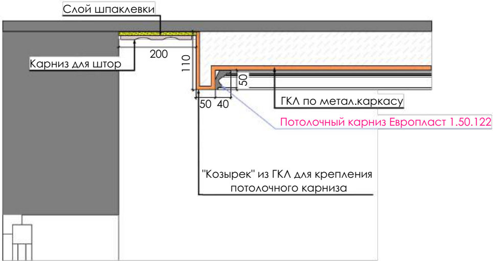
Узел 1. Ниша для карниза
