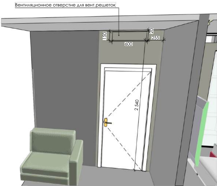
Узел 3. Вентиляционные отверстия в кабинете
