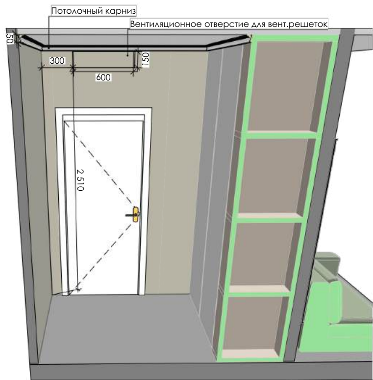
Узел 1. Вентиляционные отверстия в спальне
